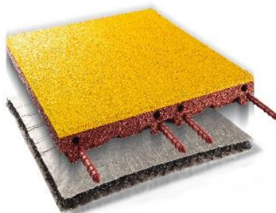
EPDM- rubbertegel (met kunststofmat)
